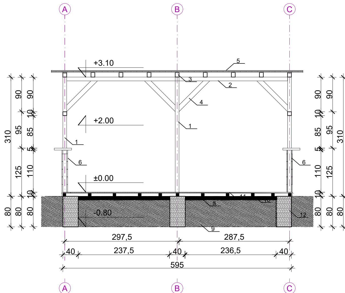
PRESJEK 1-1
