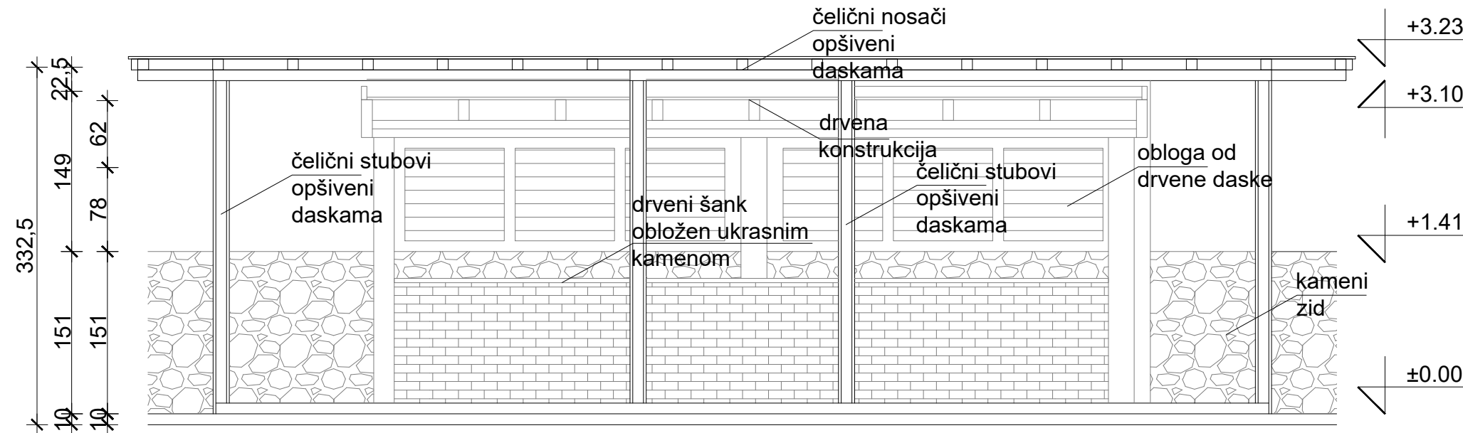
JUGO - ZAPADNA FASADA
