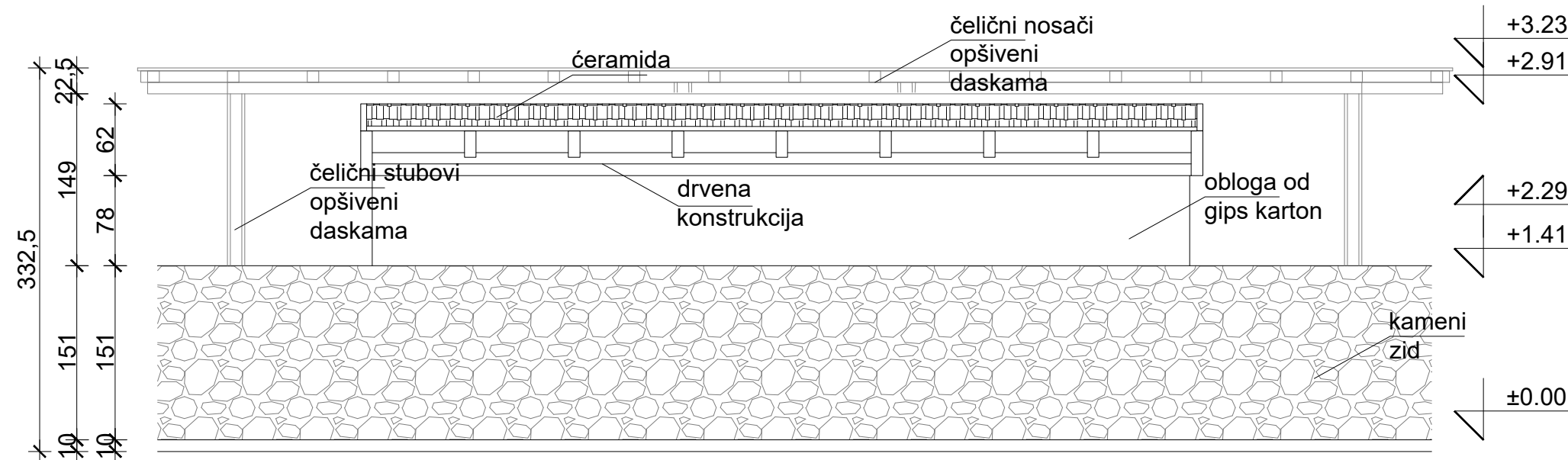
SJEVERO - ISTOČNA FASADA
