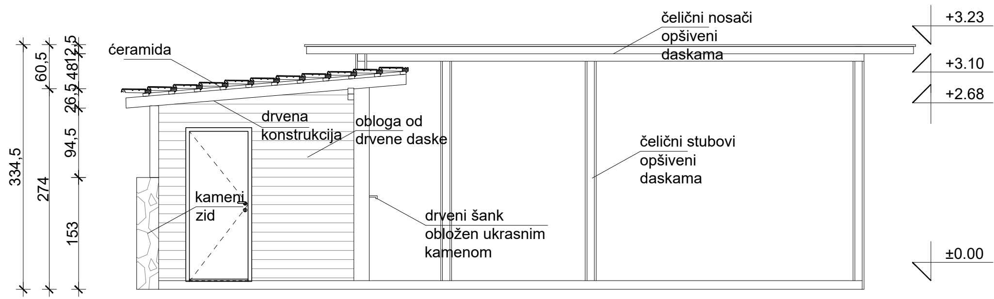
SJEVERO - ZAPADNA FASADA
