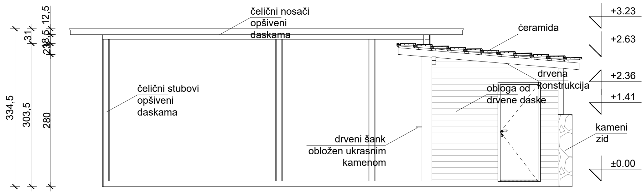
JUGO - ISTOČNA FASADA
