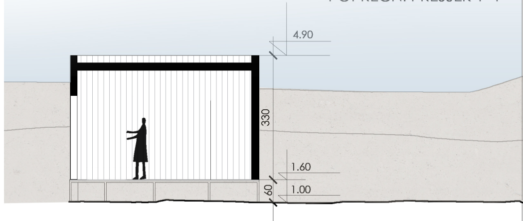
POPREČNI PRESJEK 1'-1'
