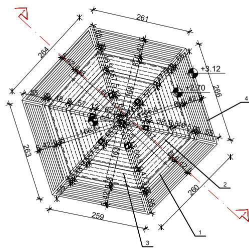
OSNOVA KROVNE KONSTRUKCIJE
