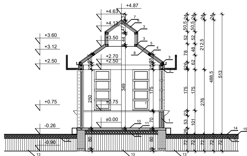
PRESJEK 1-1
