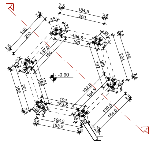
OSNOVA TEMELJA
