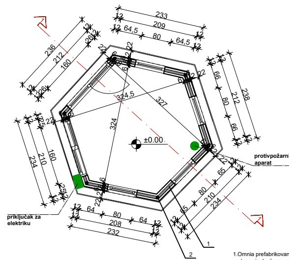
OSNOVA PRIZEMLJA
