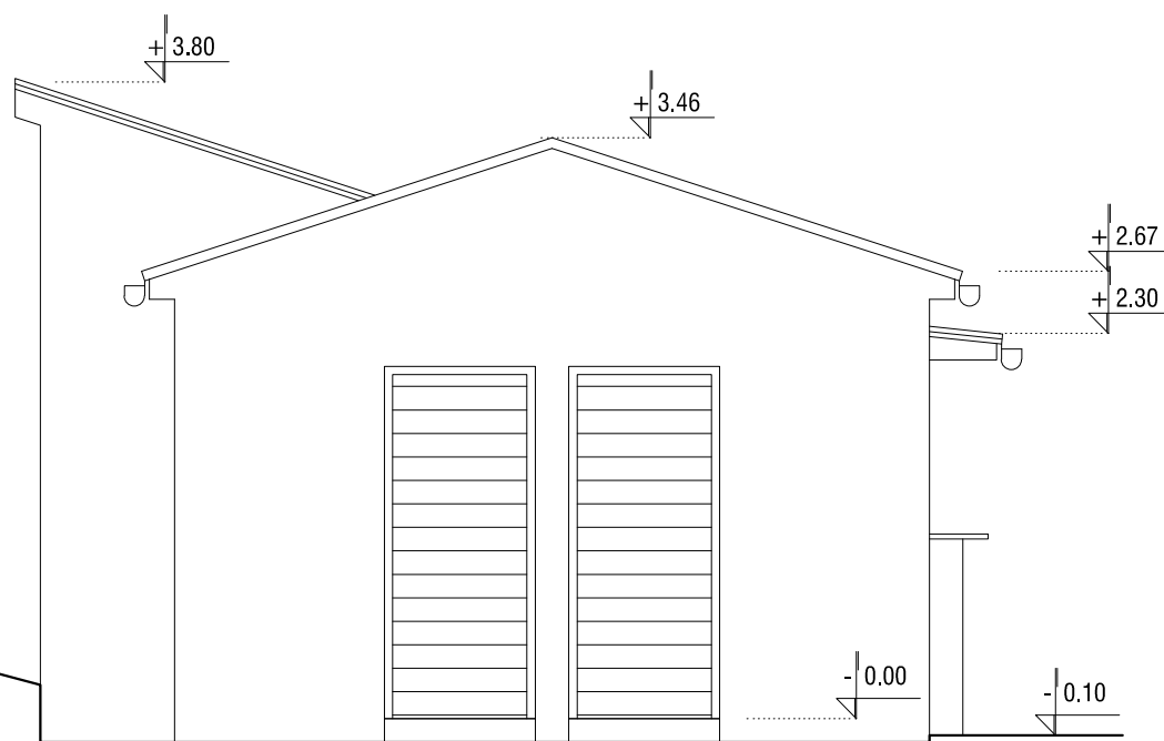
ZAPADNA FASADA
