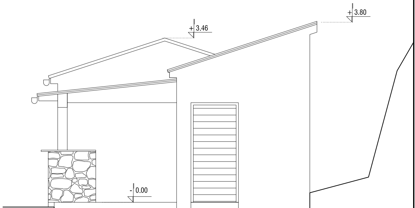
ISTOČNA FASADA
