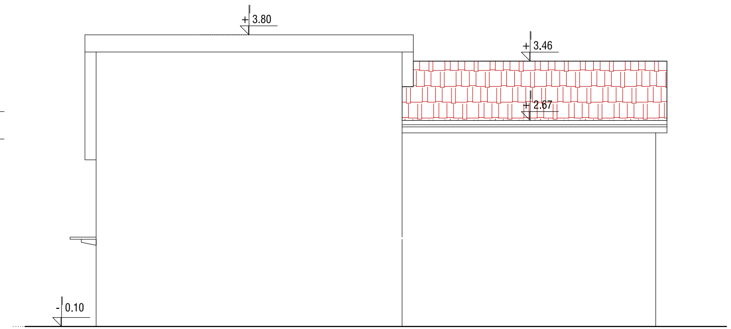
SEVERNA FASADA
