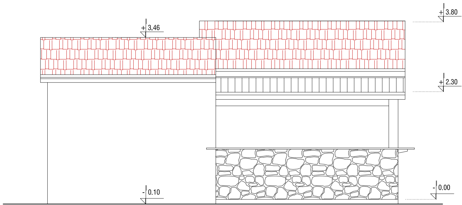
JUŽNA FASADA
