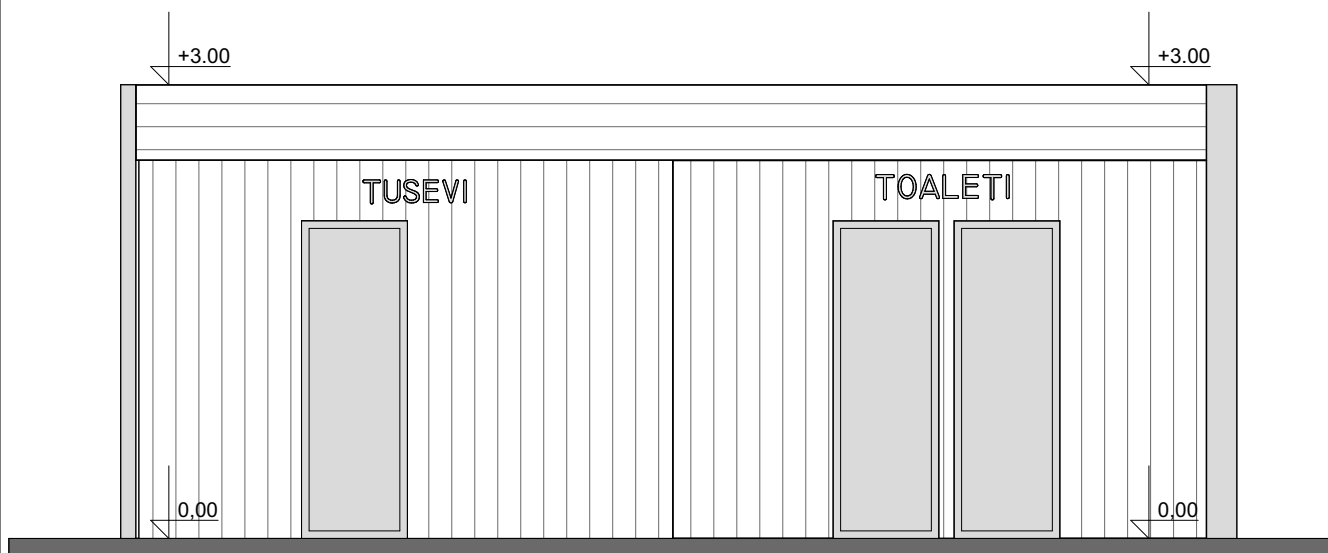
FASADA 1
