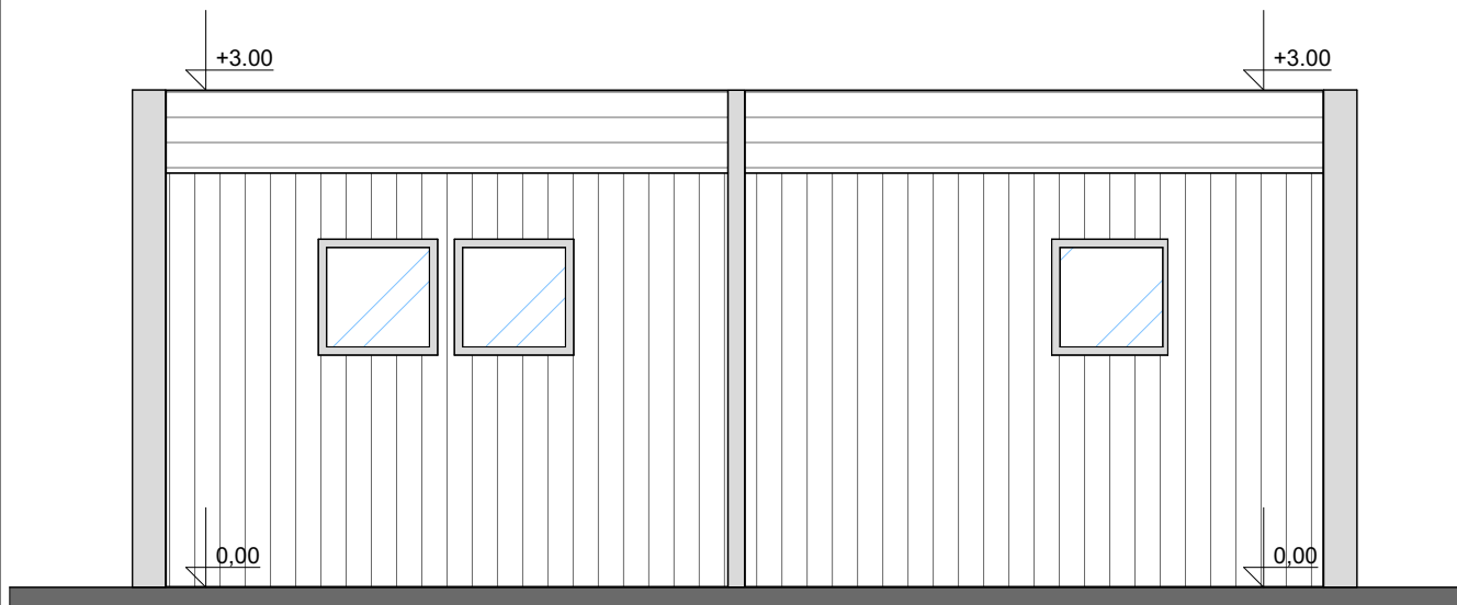
FASADA 2
