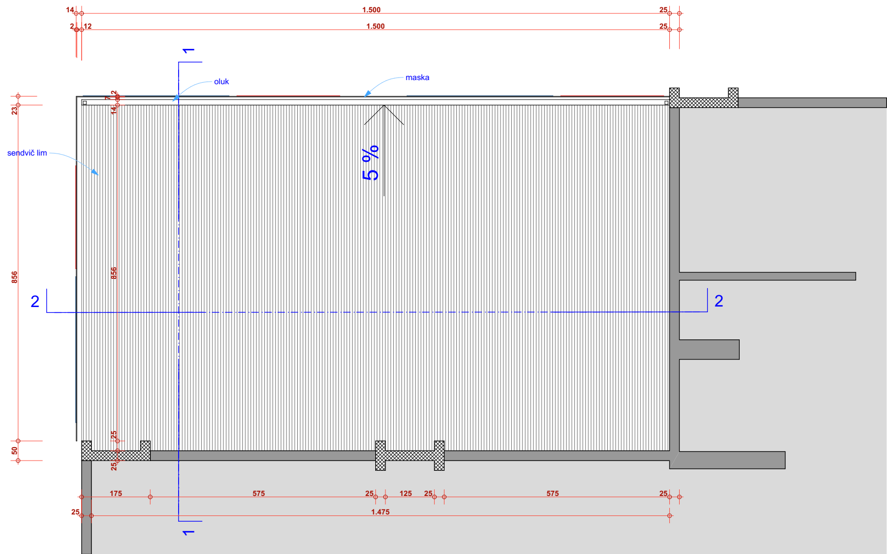
OSNOVA KROVA R = 1:100
