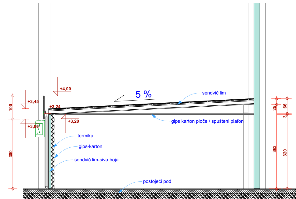
PRESJEK 1-1 R = 1:100
