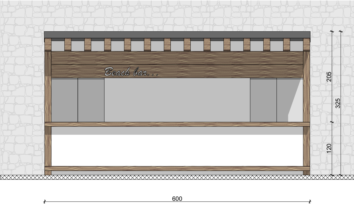
ZAPADNA FASADA
