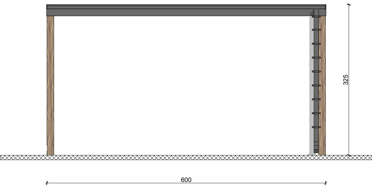
ISTOČNA FASADA
