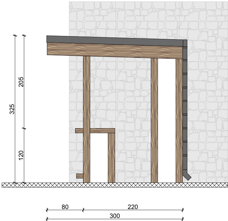
JUŽNA FASADA
