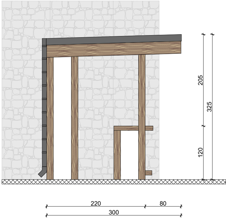
SJEVERNA FASADA
