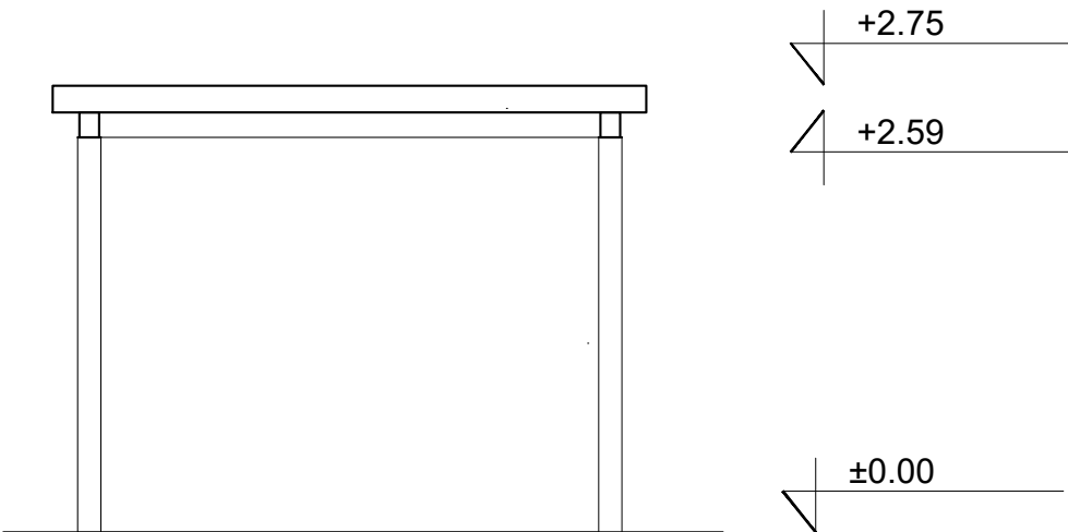
BOČNI IZGLED
